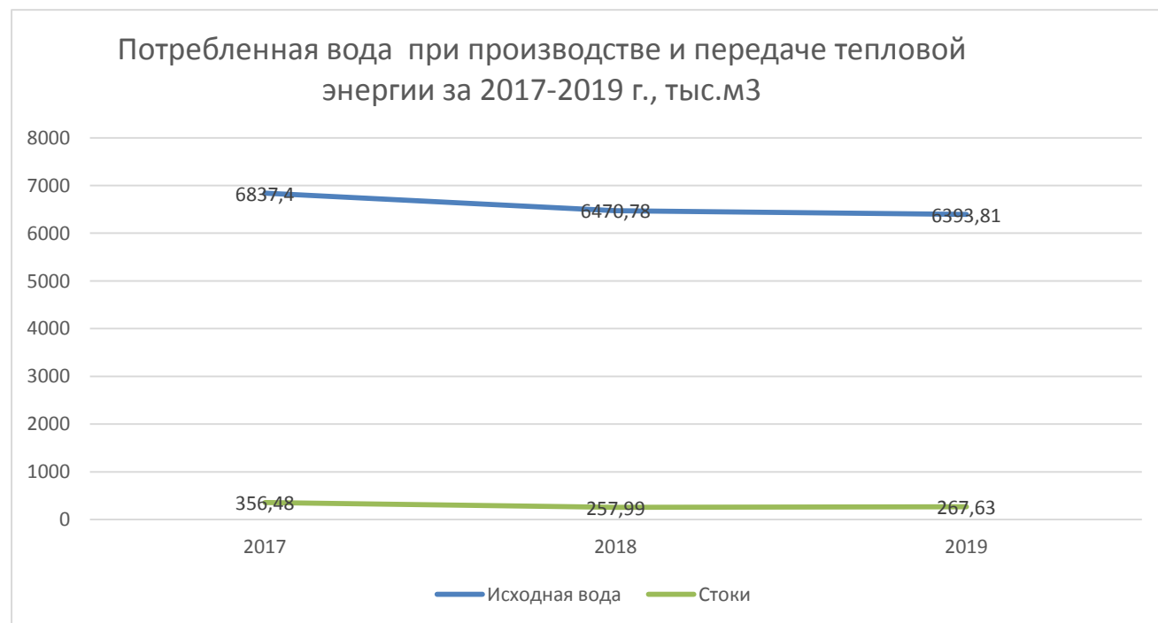
График 2.5.2. - Потребленная вода при производстве и передаче тепловой энергии за 2017-2019 г., тыс.м 3
